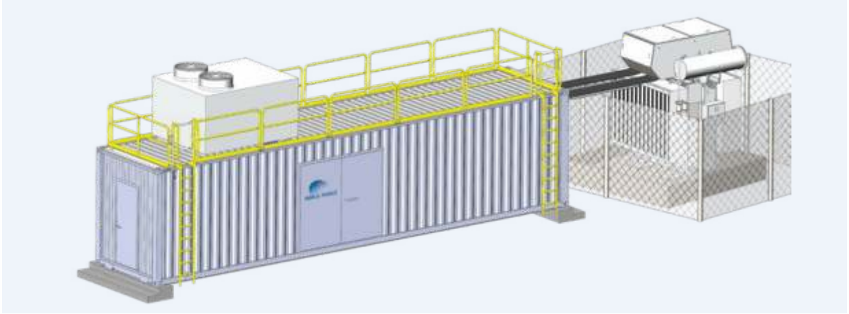
Merus ESS - tip 2: Konteynere entegre edilmiş depolama ve PCS. Yardımcı için açık güç trafosu
